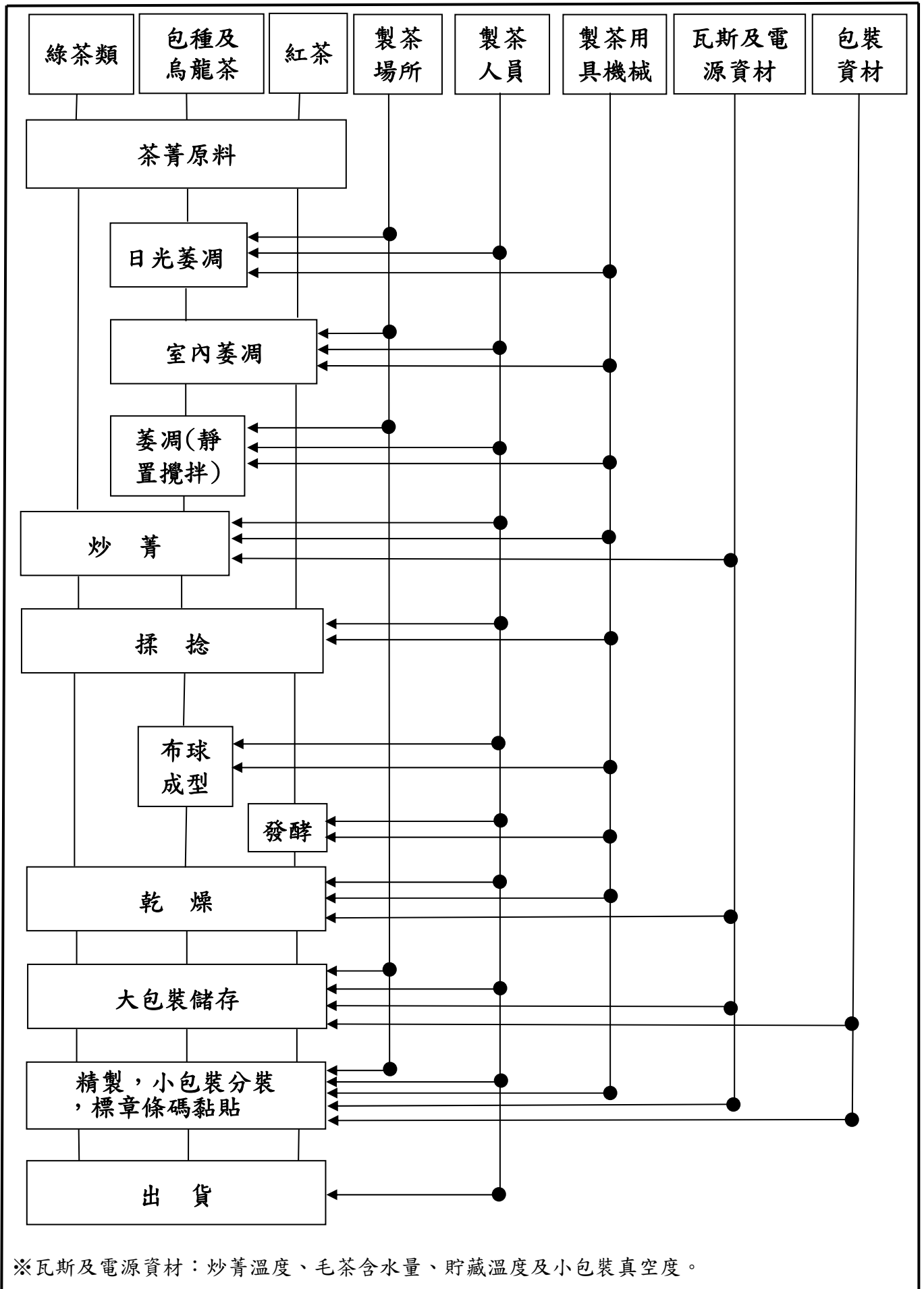
(二) 有機茶加工製造流程圖
